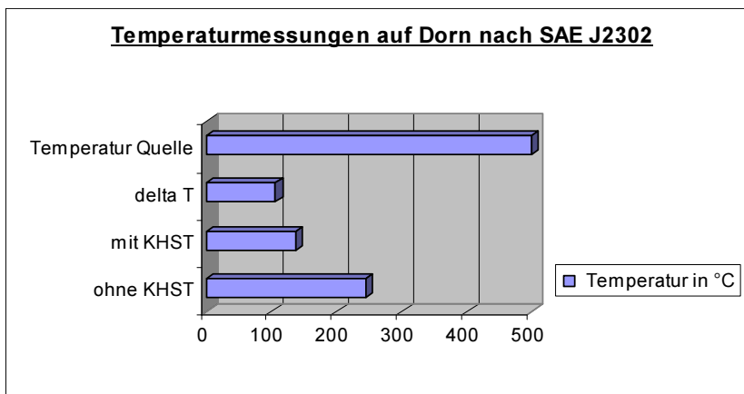
Labormessung einer Hitzeschutztasche (exemplarisch)
